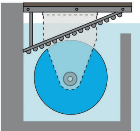
Unterflur-Rollladen mit Lamellen in PVC Solar mit Treppenanschnitt.
